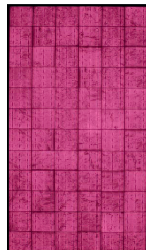
Stesso modulo FV curato con APID
