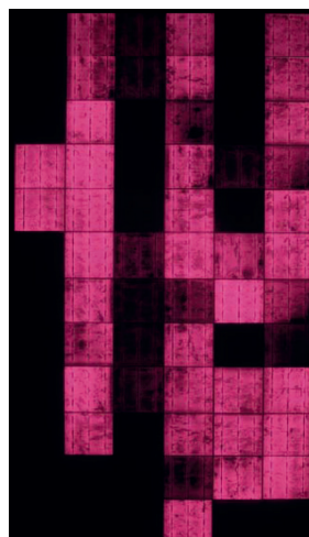
Modulo FV affetto da PID
